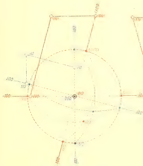
7. Пирротит.
